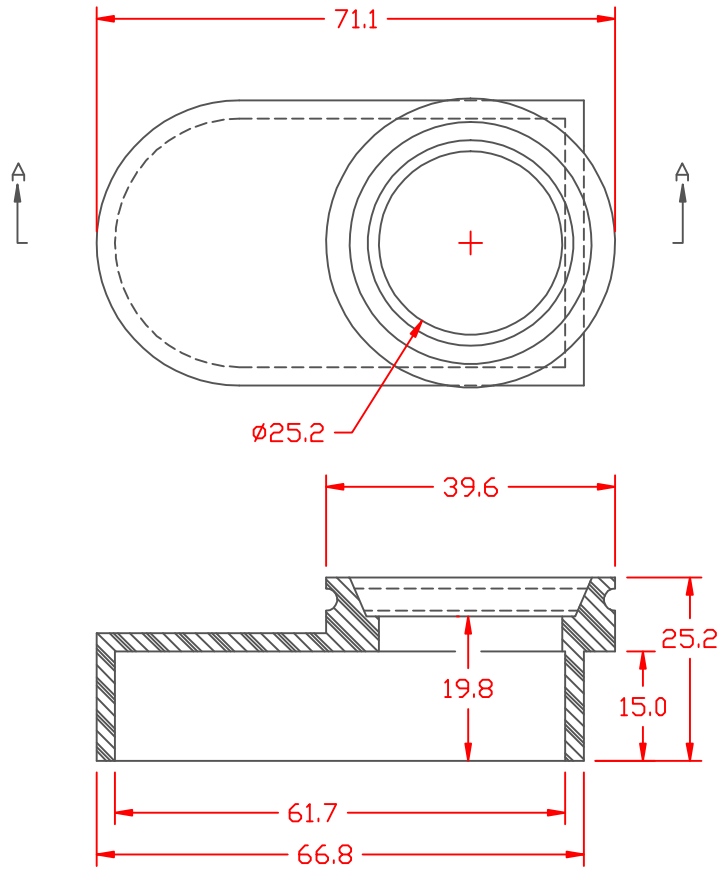
SECTION A-A
