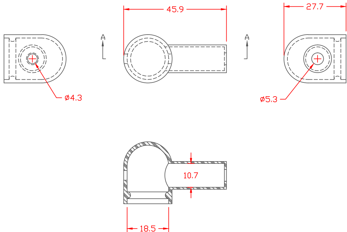
SECTION A-A
