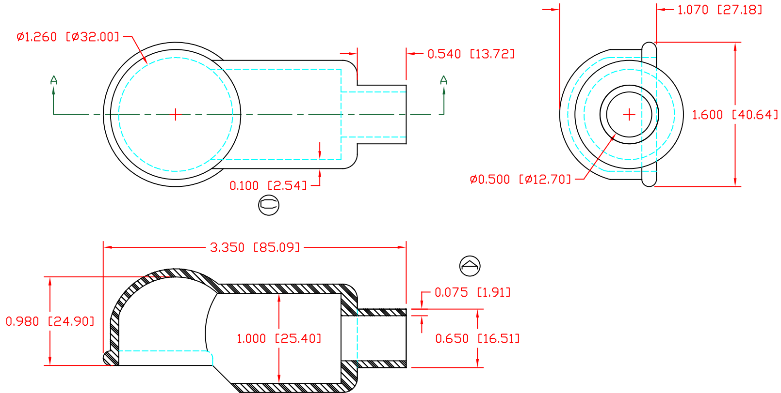
SECTION A-A
