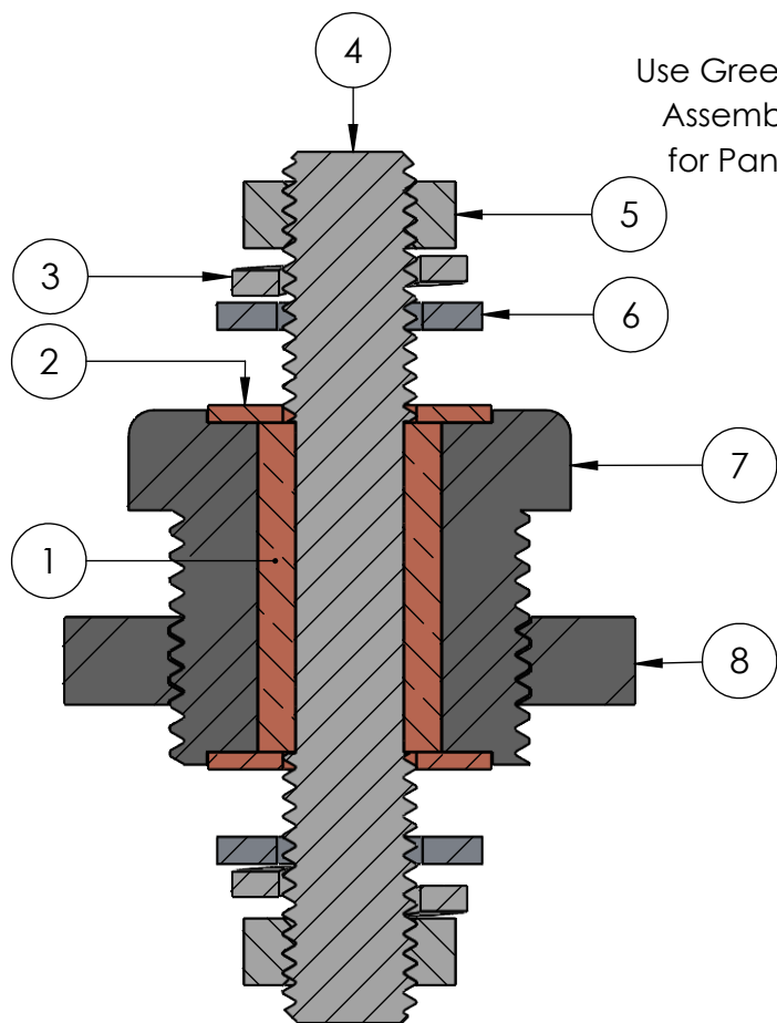
SECTION A-A
