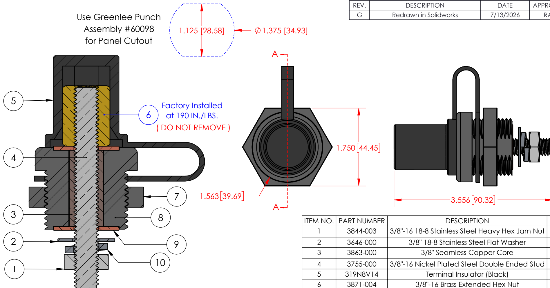
SECTION A-A
