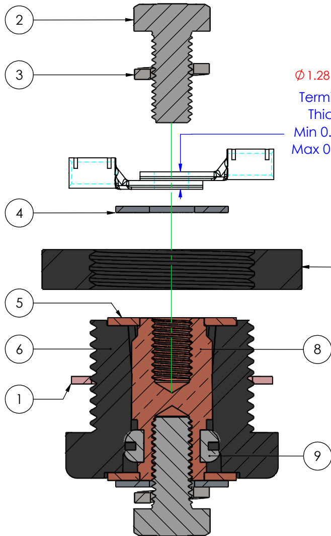
SECTION A-A
